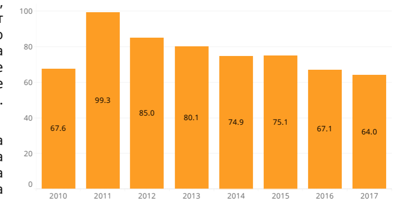
Слика 32: Годишно средно ниво на ситни честички во градовите (µg/m3)
